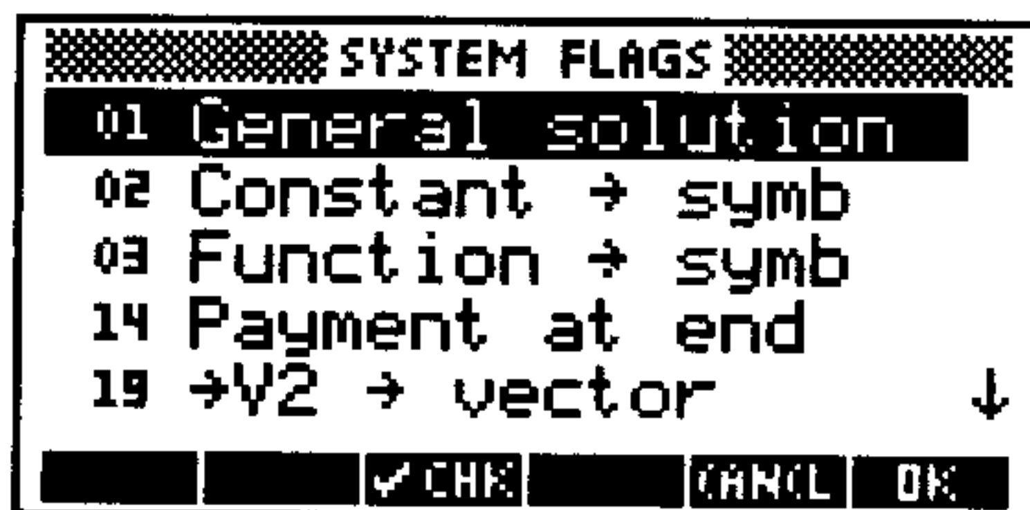
The Flag Browser
